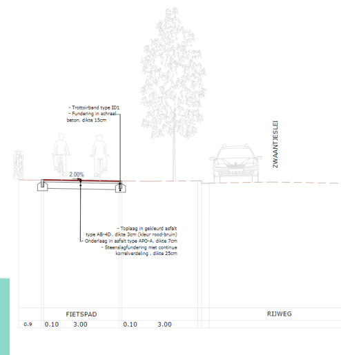
TYPEDWARSPROFIEL A
